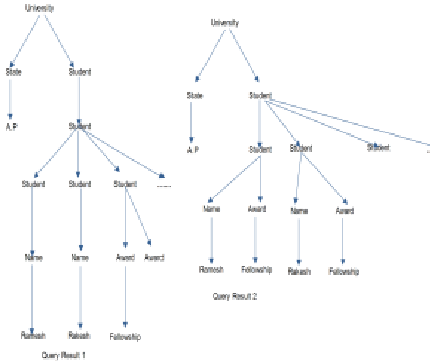
A).Sub Tree
